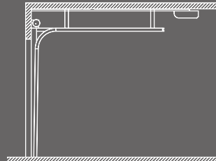
Направляющие типа NH Направляючі типу NH
